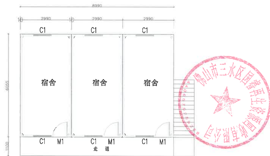
二层平面参考布置图
