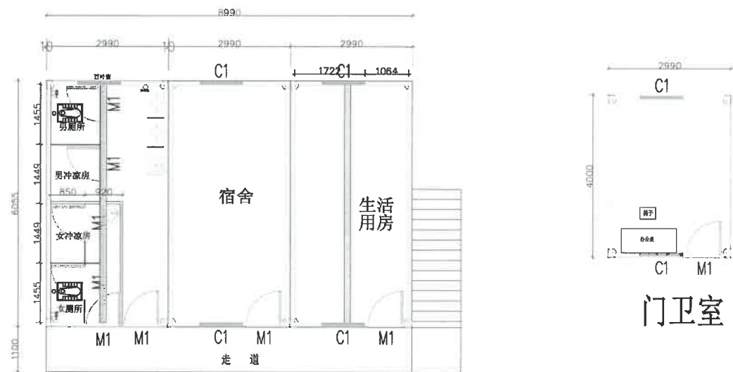
一层平面参考布置图
