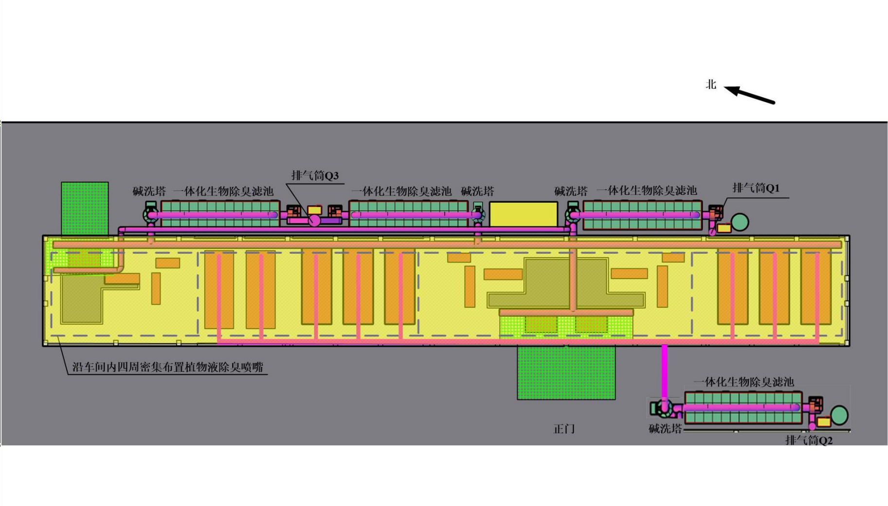
图4 项目恶臭气体收集方案效果图 (a)
